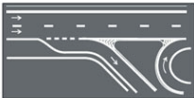
Ordenação de movimentos em trevos com alças e faixas de aceleração / desaceleração
