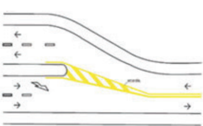
ACOMODAÇÃO PARA INÍCIO DE CANTEIRO CENTRAL
