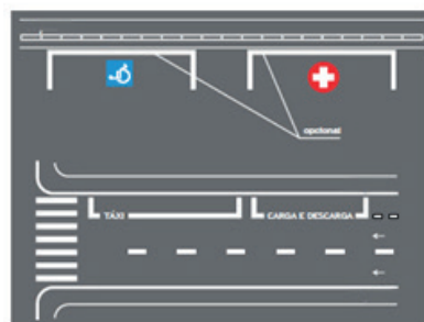
Estacionamento paralelo ao meio-fio
