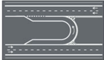
Ordenação do movimentos em retornos com faixa adicional para o movimento
