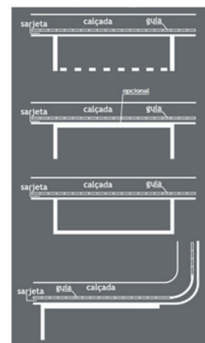
Marca delimitadora de estacionamento regulamentado. Paralelo ao meio-fio: linha simples contínua ou tracejada
